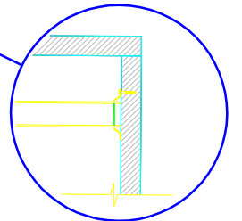
DETALLE 1:20
