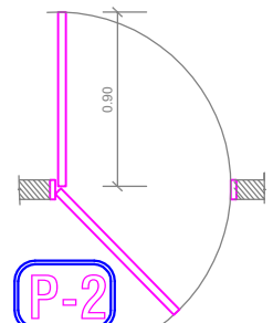
PUERTA VAIVÉN PERFILES ACERO INOXIDABLE MARCO: ACERO INOXIDABLE UNIDAD: UNA (1)
