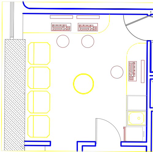
PLANTA ESTAR DE MEDICOS 1:20
