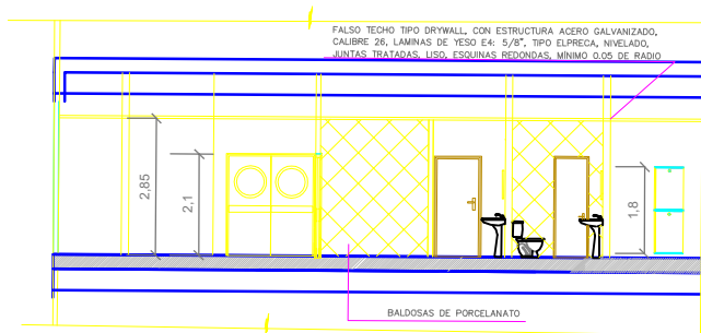
CORTE E-E
