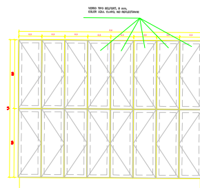
FACHADA 1:20
